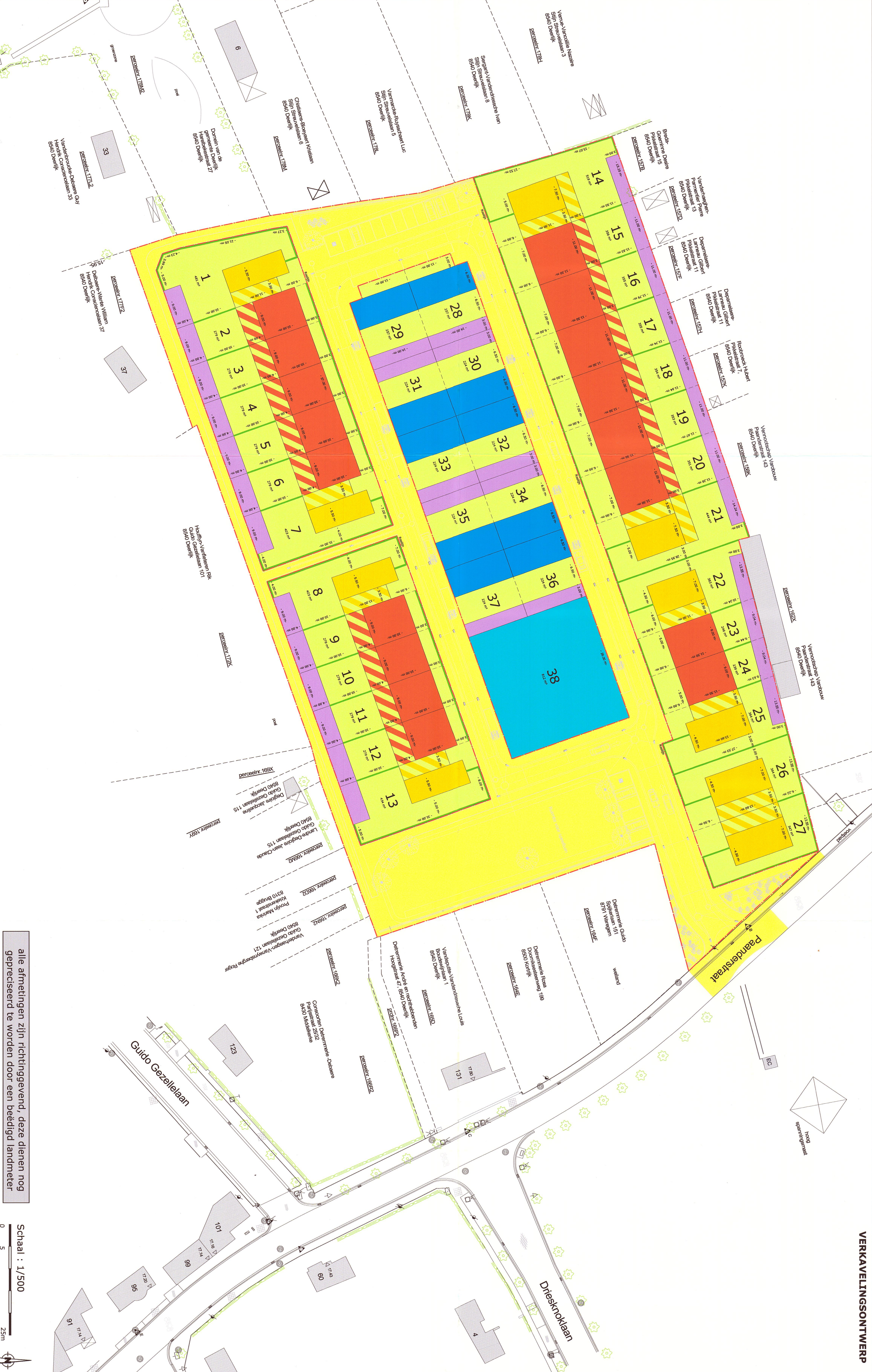
Schaal: 1/500
